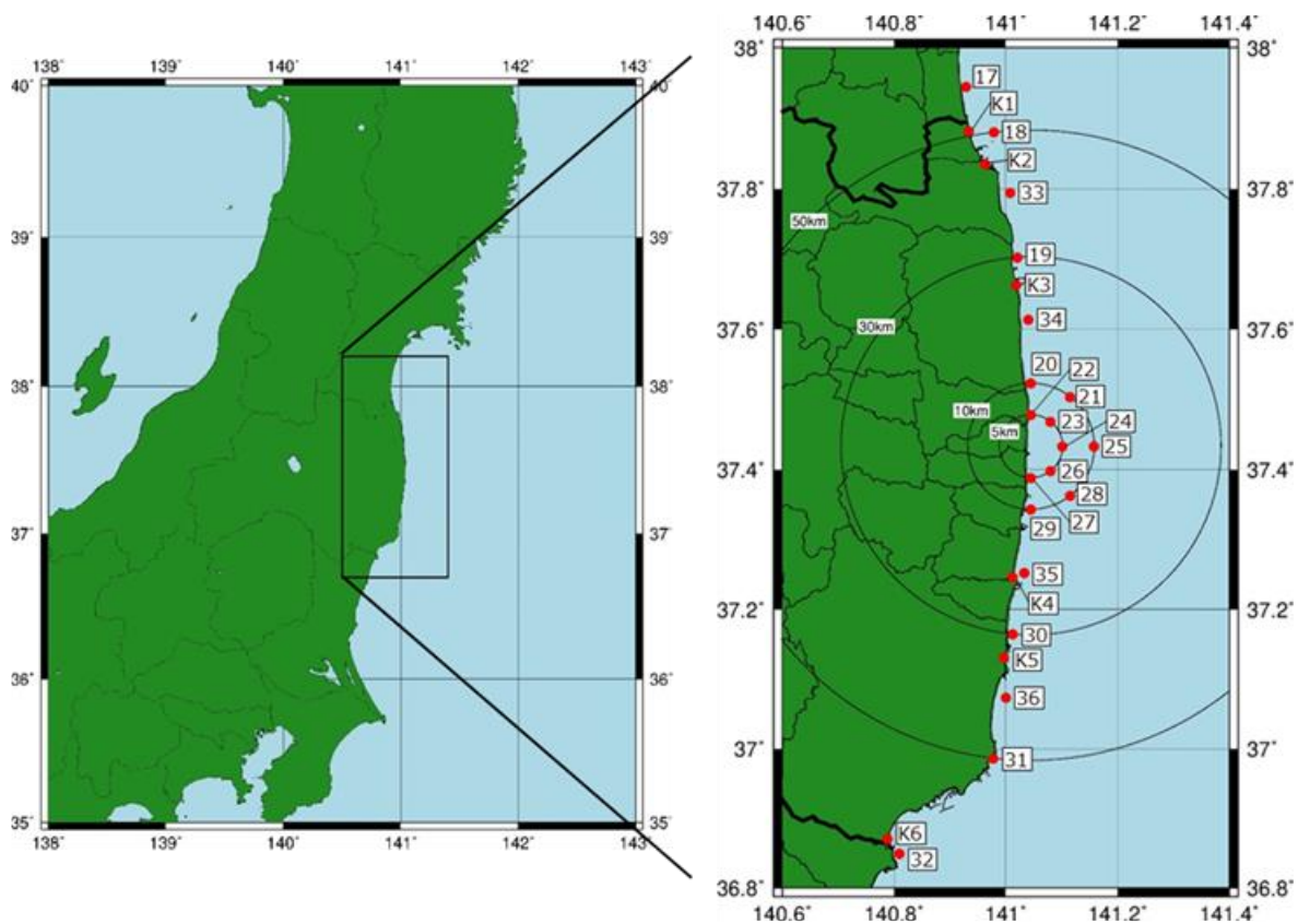
図 海水中のトリチウムの測点 (ALPS 処理水放水口予定箇所から 3 km 圏外)
