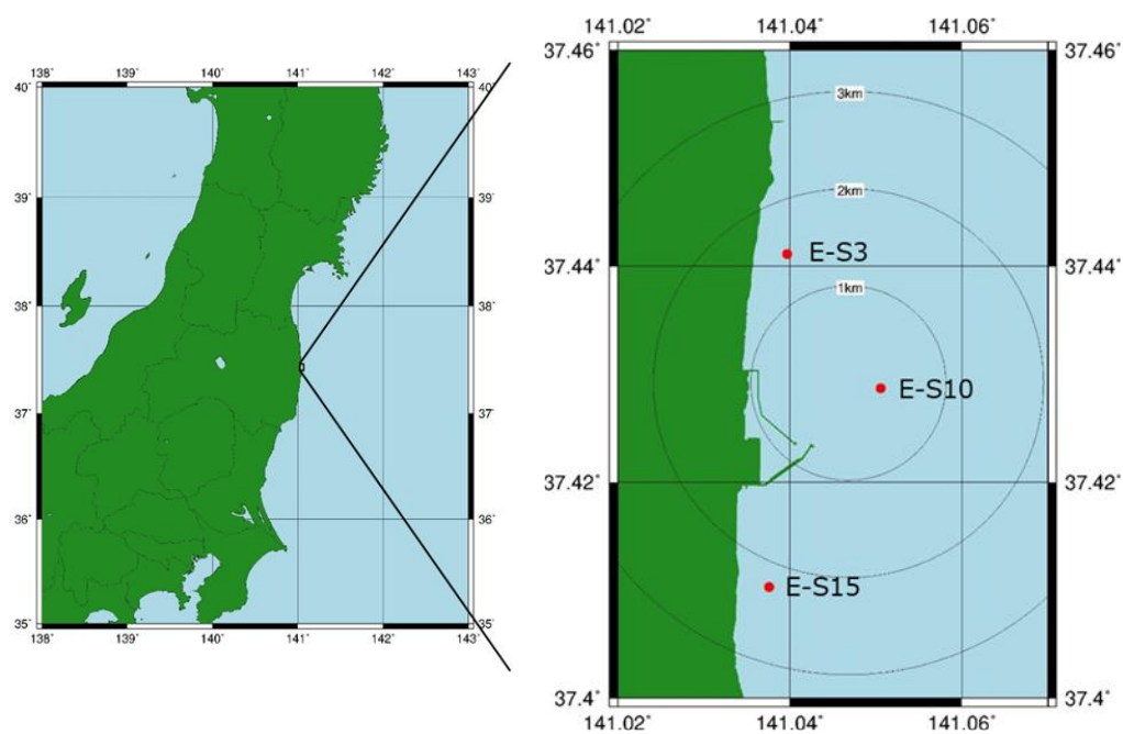
図 1 海水中の主要 7 核種の測点
